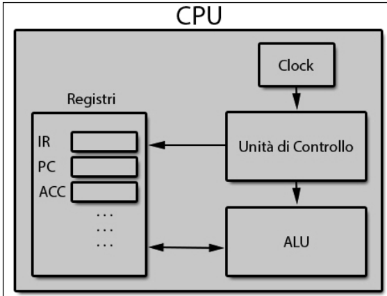
Figura 1.4 Struttura logica di una CPU.
