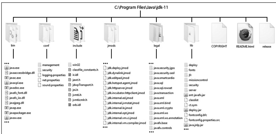
Figura 1.9 Struttura ad albero del JDK 11 a 64 bit creata in un sistema Windows.
