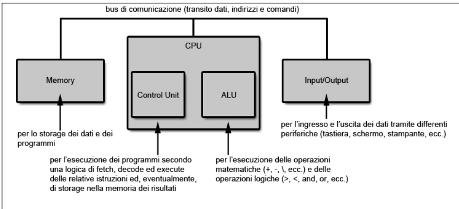
Figura 1.3 Architettura semplificata di un computer, basata sul modello di von Neumann.
